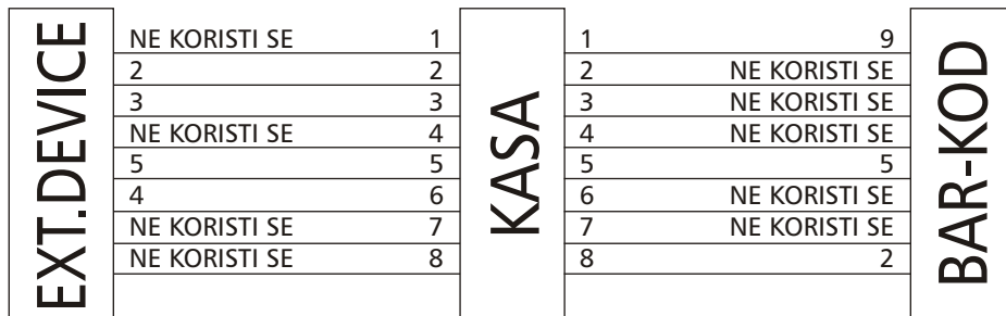
Šema povezivanja PC-a, Bar Code-a i Kase
