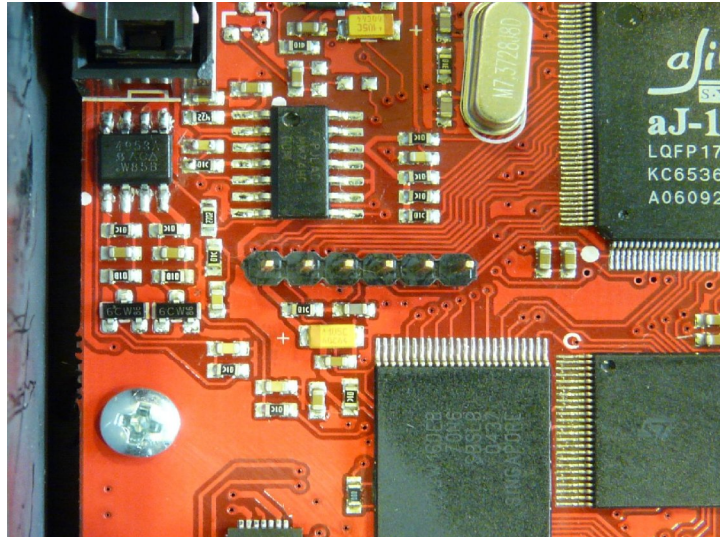
Slika 4. – konektor za programiranje
