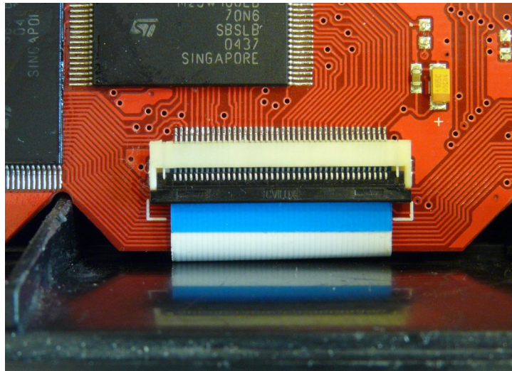
Slika 2. – konektor za povezivanje fiskalne memorije
