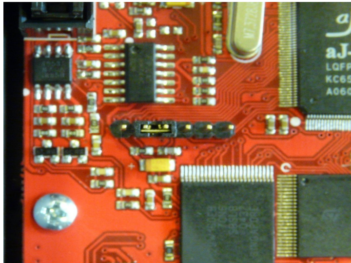
Slika 5. – konektor za programiranje sa zaštitnim kratkospojnikom
